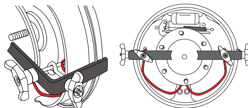
2007 SILVERADO HUB
